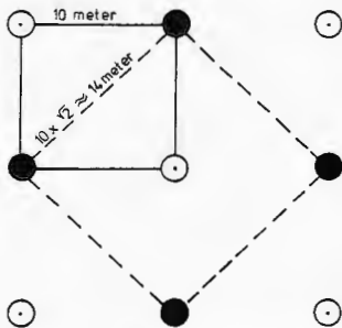
Figur 3. Justering av 10-metersförband till 14-metersförband. Man erhåller lätt 14 m mellan ekarna om man planerar för diagonalförband vid huggningarna.
